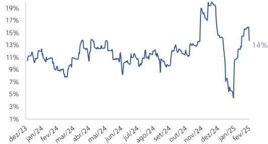
Volatilidade [2]
